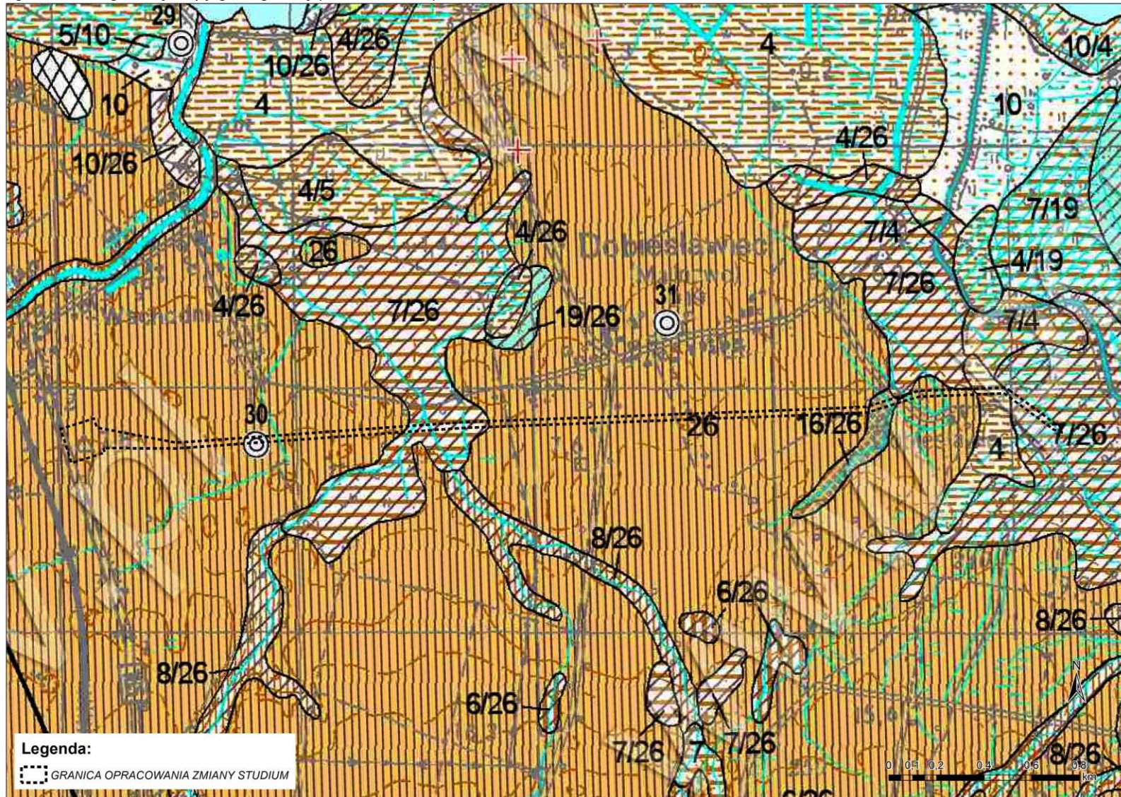
Rysunek 6 Fragment szczegółowej mapy geologicznej (skala 1:50 000).
